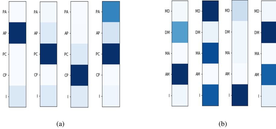
图 3: 在图 1 中对 1 \times 1 卷积滤波器 W_{\phi}^i ( i : 层索引) 应用 softmax 函数后，我们可视化了 DBLP（左侧）和 IMDB（右侧）数据集中邻接矩阵（边类型）的注意力分数。(a) 分别表示每条边为 (论文-作者)、(作者-论文)、(论文-会议)、(会议-论文) 以及单位矩阵。(b) IMDB 数据集中的边分别表示 (电影-导演)、(导演-电影)、(电影-演员)、(演员-电影) 以及单位矩阵。
